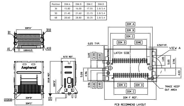
Drawing for mini SAS
