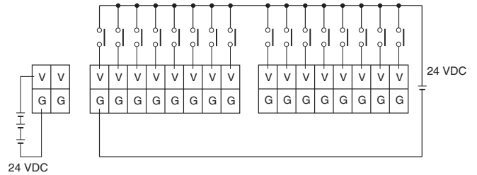
G70V-SID16P-1-C16
