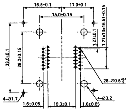
SOP IC51-334-1.KS-6411 (24 Pins) SOP IC51-0282-334-1 (28 Pins)
