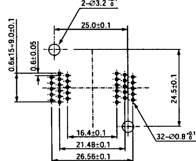
SSOP IC51-0322-910 (32 Pins)
