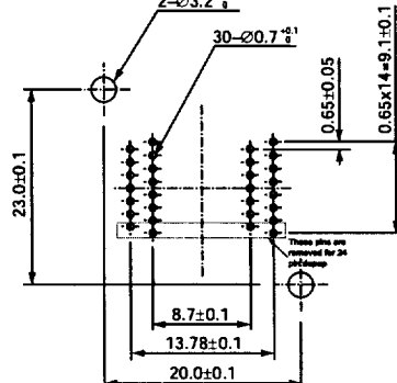
SSOP IC51-0302-755 (30 Pins)
