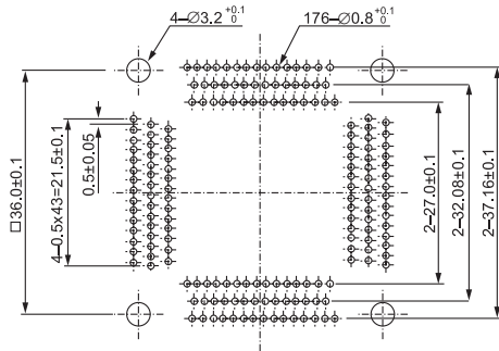
IC51-1764-1505 (176 Pins)
