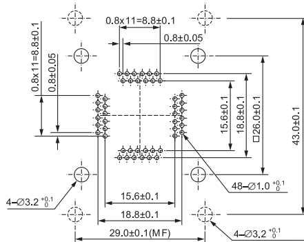
IC51-0484-081 (48 Pins)
