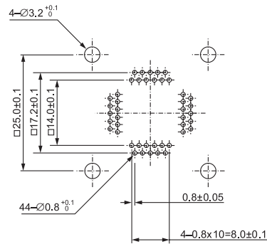
IC51-467-KS11787 (44 Pins)
