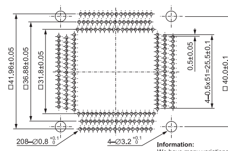
IC51-2084-1052-* 2) (208 Pins)
