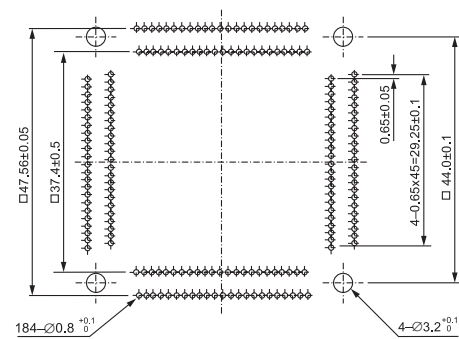
IC51-1844-1148-1 (184 Pins)
