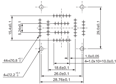
IC51-0444-615 (44 Pins)
