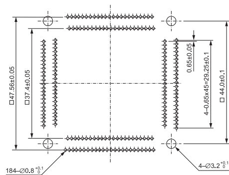
IC51-1844-1541 (184 Pins)
