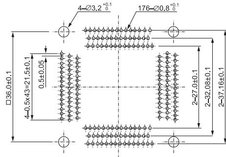
IC51-1764-1505 (176 Pins)
