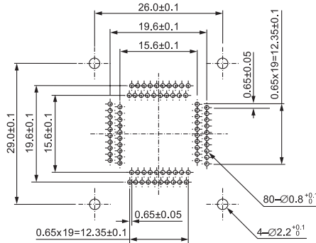
IC51-0804-956-2 (80 Pins)
