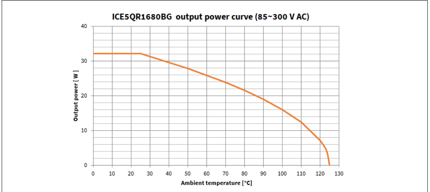
图 31 ICE5QR1680BG 的输出功率曲线, V_{IN}=85\sim 300 V_{AC} ; P_{Out}=f(T_a)
