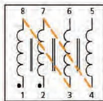
CM5740Z241B-10, CM 45 Array
