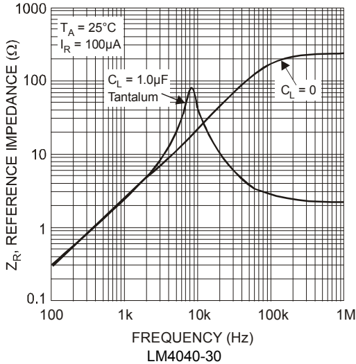
LM4040-30
