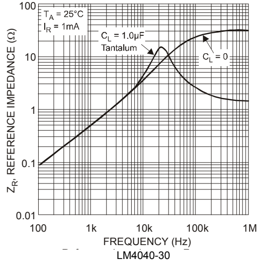
LM4040-30
