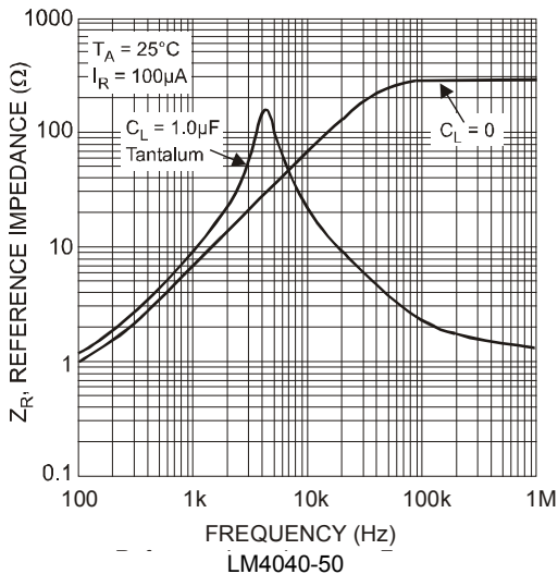
LM4040-50
