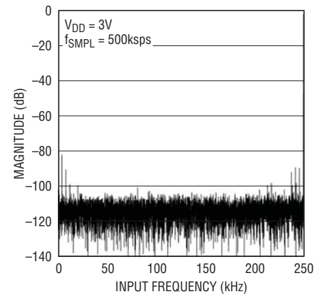
248kHz Sine Wave 8192 FFT Plot
