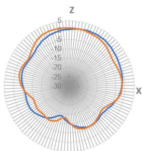
— 1575 MHz — 1602 MHz
