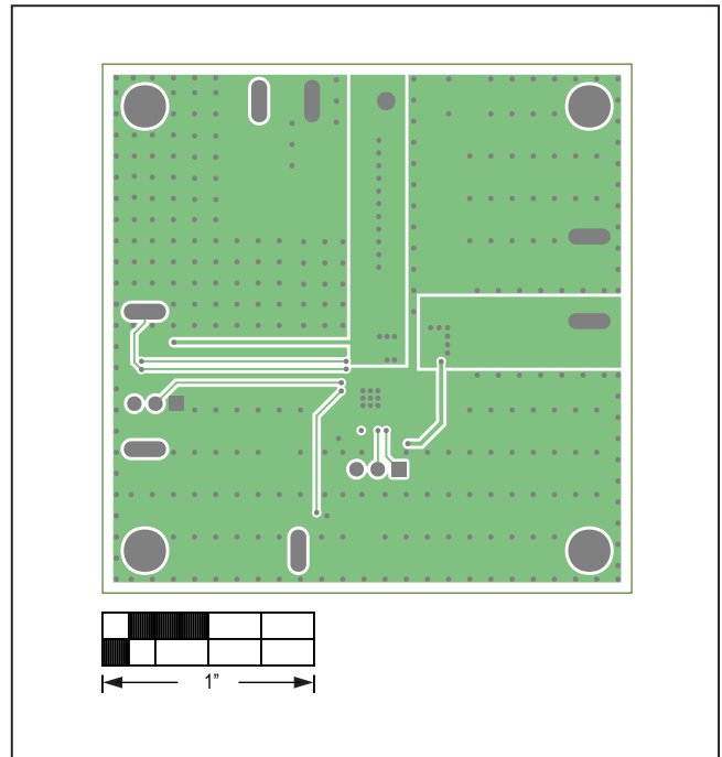
L3 PWR
