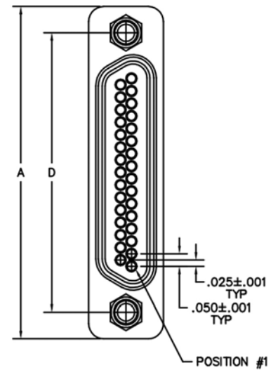
RECEPTACLE
