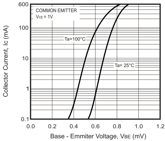
Fig.5 - I_c — V_{BE}
