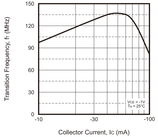
Fig.6 - f_T — I_C
