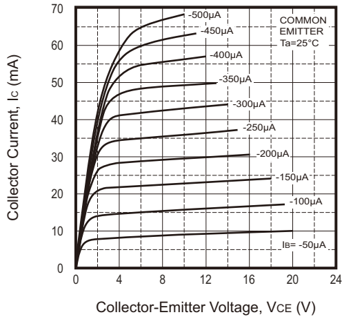
Fig.1 - I_C - V_{CE}
