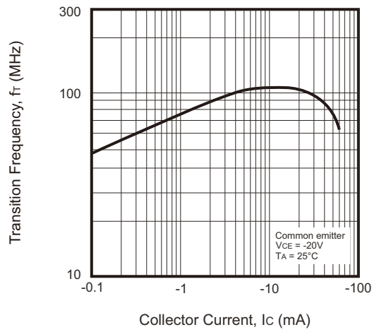
Fig.6 - f_r - I_c
