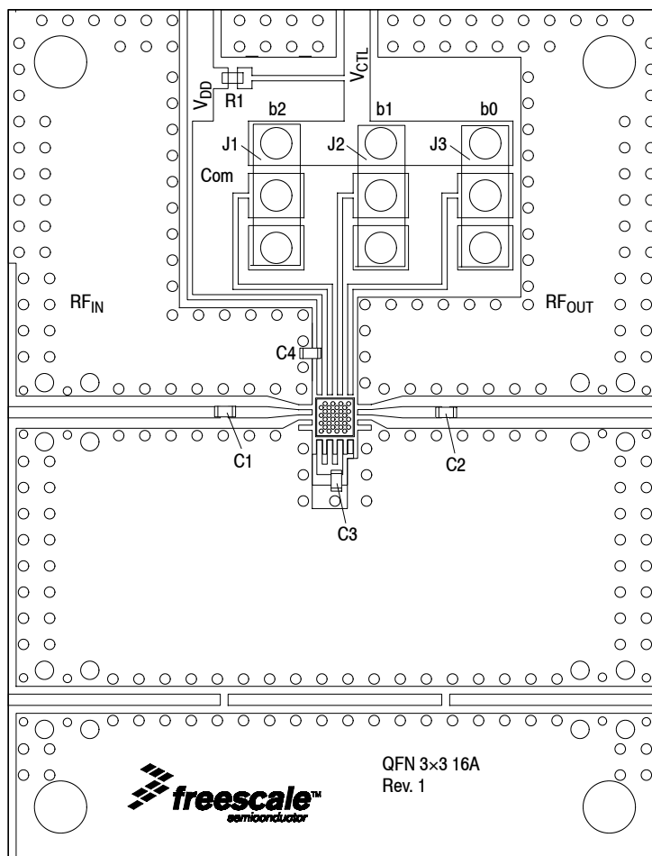
PCB actual size: 1.25" × 1.62".
