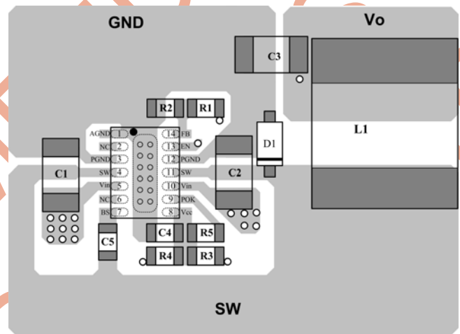
Top Layer
