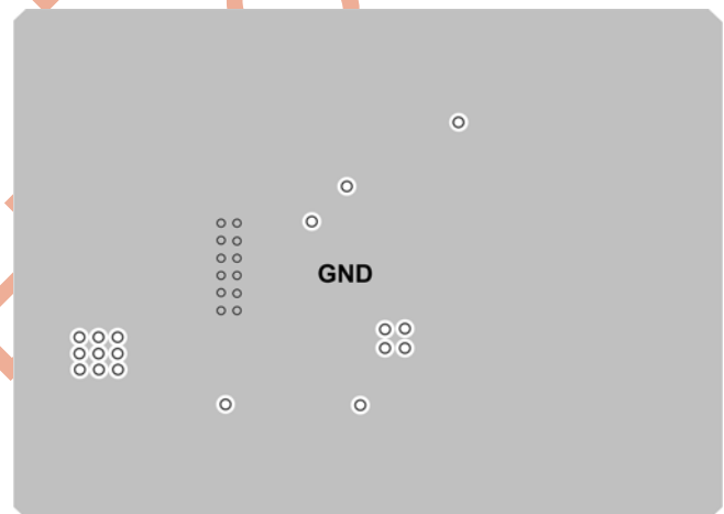
Inner Layer1
