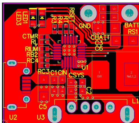
Top Layer
