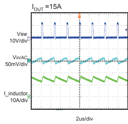
Input Ripple
