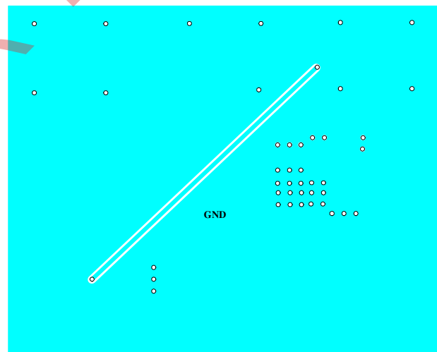
Inner2 Layer
