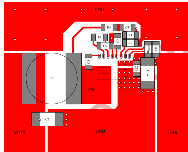
Top Layer
