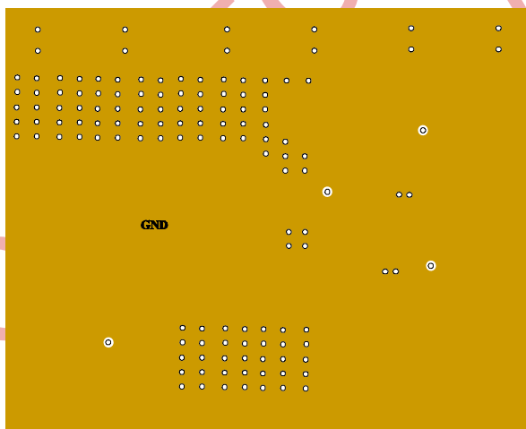
Inner1 Layer
