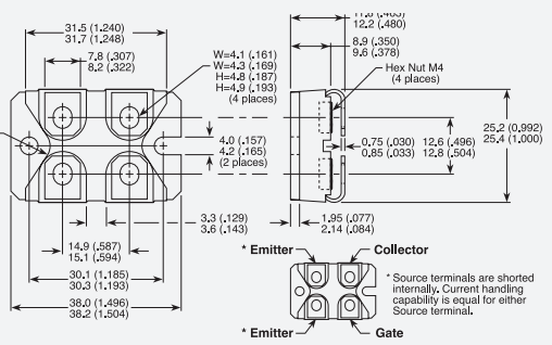
ISOTOP® or SOT-227
