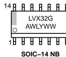
SOIC-14 NB
