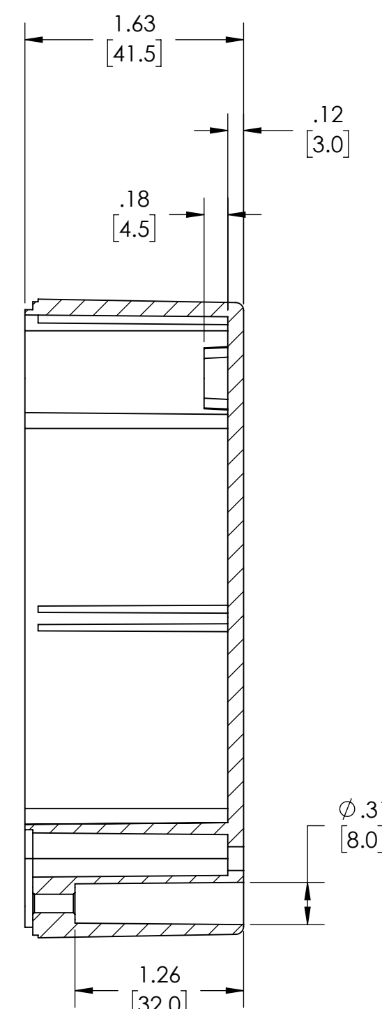
SECTION A-A
