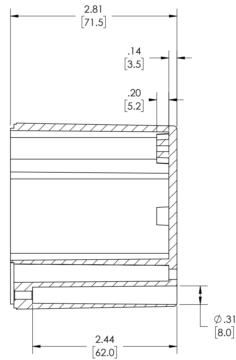
SECTION A-A
