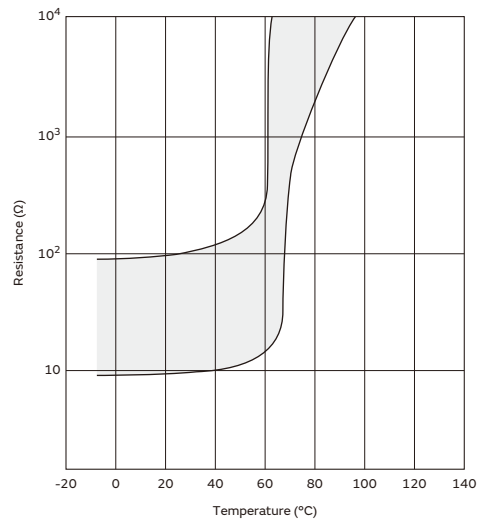
PTF_04BG471Q Type
