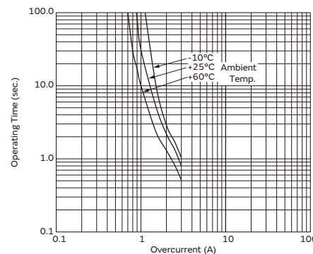
PTGL06AR0R8M1B51B0
