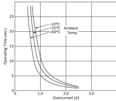
PTGL13AR100H8B72B0
