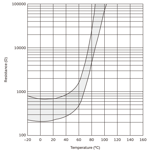
PRF18BF471Q Type
