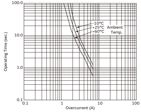
PTGL09ARR33M1B51B0
