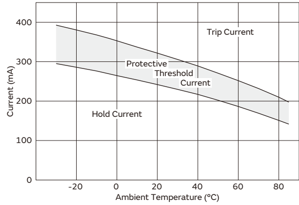
PTGL09AS3R3K4B51B0
