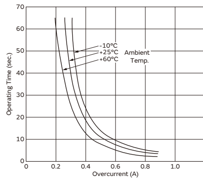
PTGL09AR250H8B52B0
