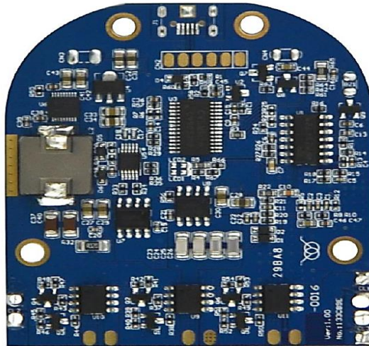
PCBA Size : 52(±0.3) * 53.5 * 4.7(±0.2) mm
