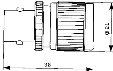
C FEMELLE - SMB MALE Étanche de panneau, à écrou
