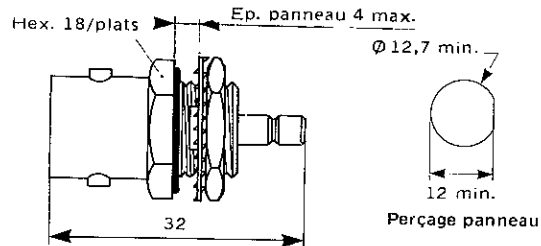
C FEMELLE - SMB MALE Étanche de panneau, à écrou
