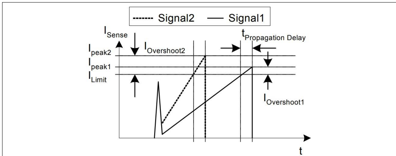
图 10 限流
