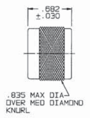
RFI385-1 SHOWN NO CHAIN/ROPE OR MOUNTING LUG
