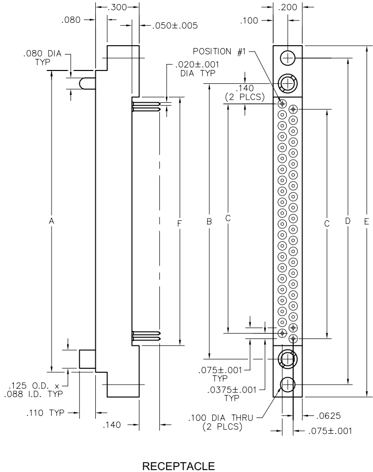
RECEPTACLE
