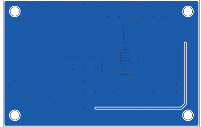
Layer 2 (Signal)
