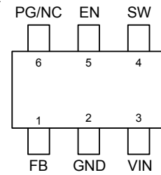
SOT-563 (FC)
