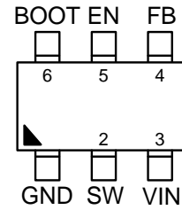
TSOT-23-6 (FC)
