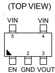
SOT-23-5
