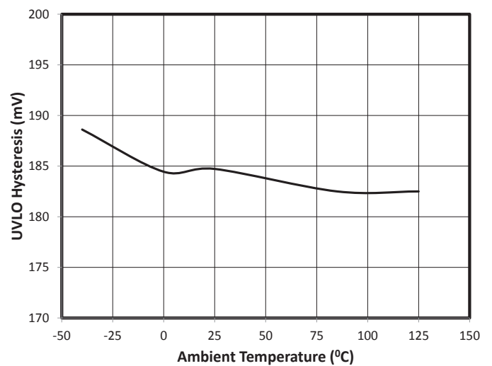
UVLO Hysteresis
