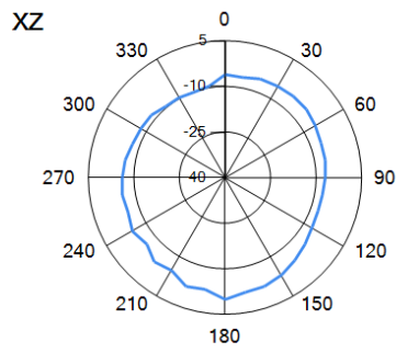
— 657MHz
