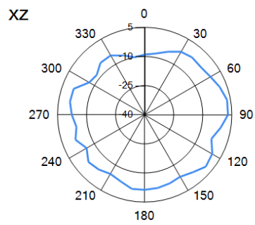
— 2.6GHz
