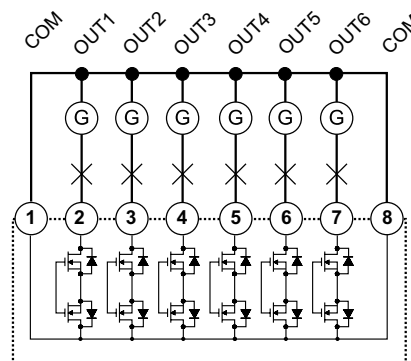
Fig. 6 M F I6 O6: opto-mosfet outputs
