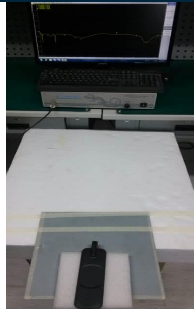
Antenna bent 90°
