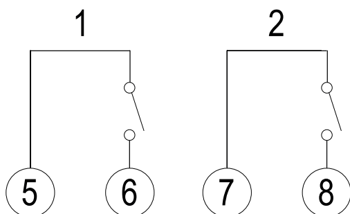
Fig. 9 Digital input 1
