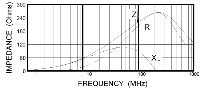
WLBD2012K2U221TP
