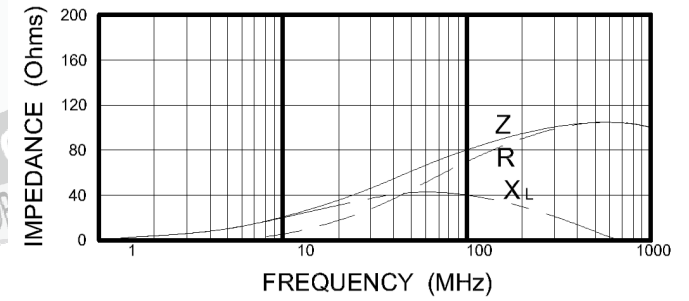
WLBD2012K2U800TP
