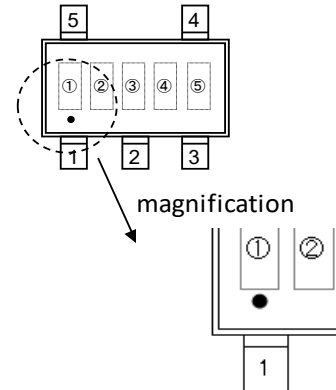
SOT-25
