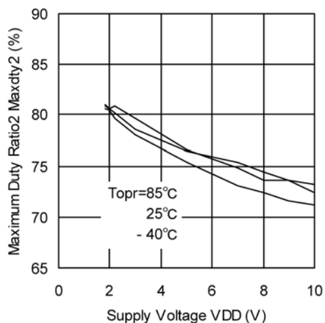
XC9505B092 (180kHz)
