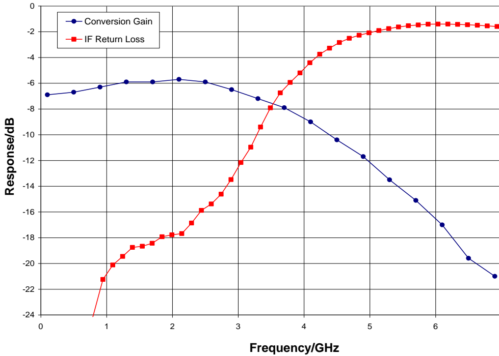
IF Bandwidth, LO = +19 dBm
