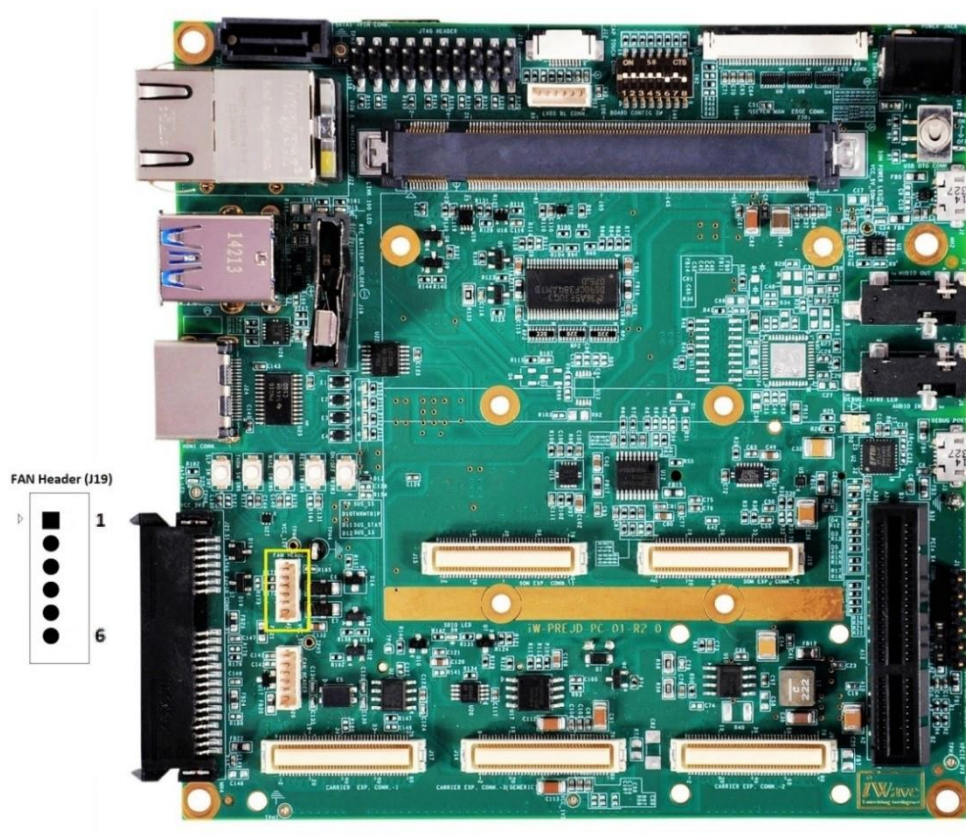
Figure 19: Fan Header
